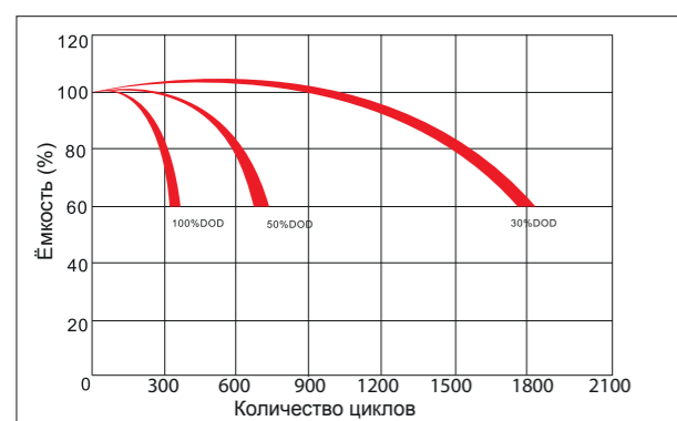
Зависимость количества циклов от глубины разряда (25°С)
